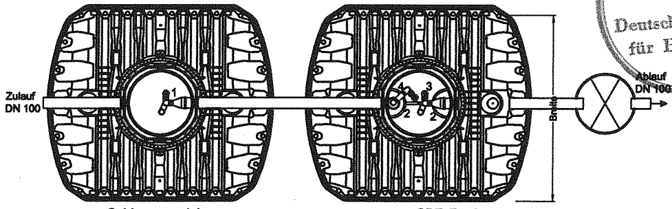
Schlamm-speicher / Puffer SBR-Reaktor
